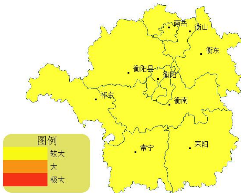
图 1 衡阳市地质灾害气象风险预警趋势图
