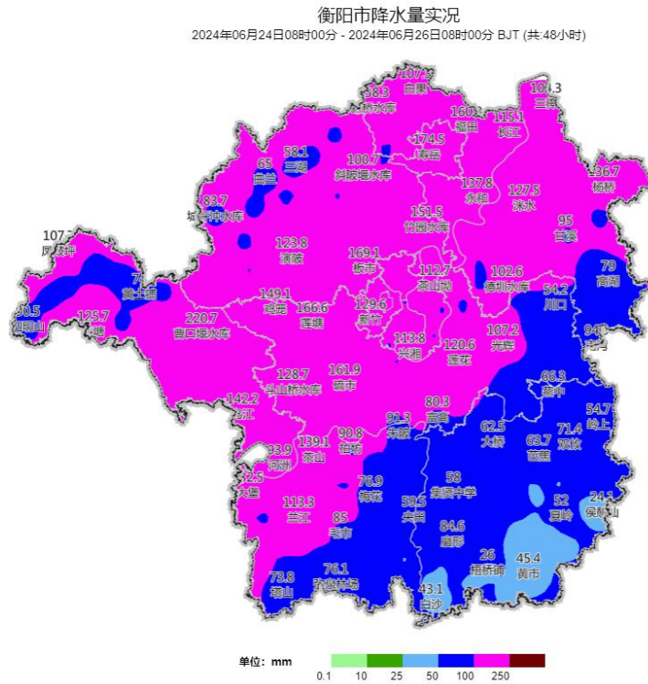
附图 2: 衡阳市地质灾害气象风险预警趋势图
